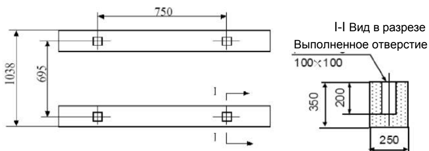
Схема фундаментного основания
